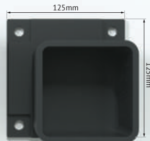
Platine au sol Floor Plate
